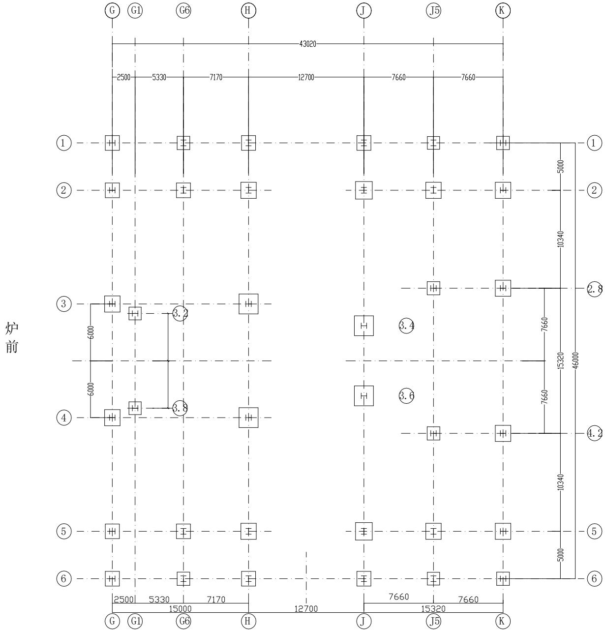
图1 锅炉平面布置示意图
