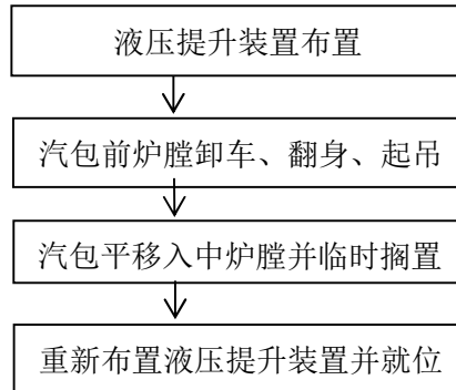
图2 锅炉汽包吊装流程图
