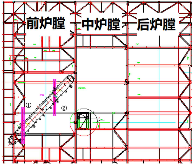
图4 汽包平移示意图-固定端头部进入中炉膛区域
