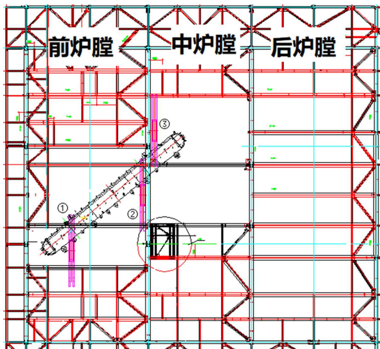
图5 汽包平移示意图-固定端换钩
