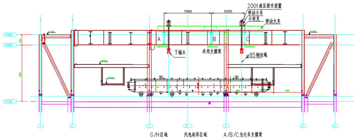
图3 液压提升装置布置示意图
