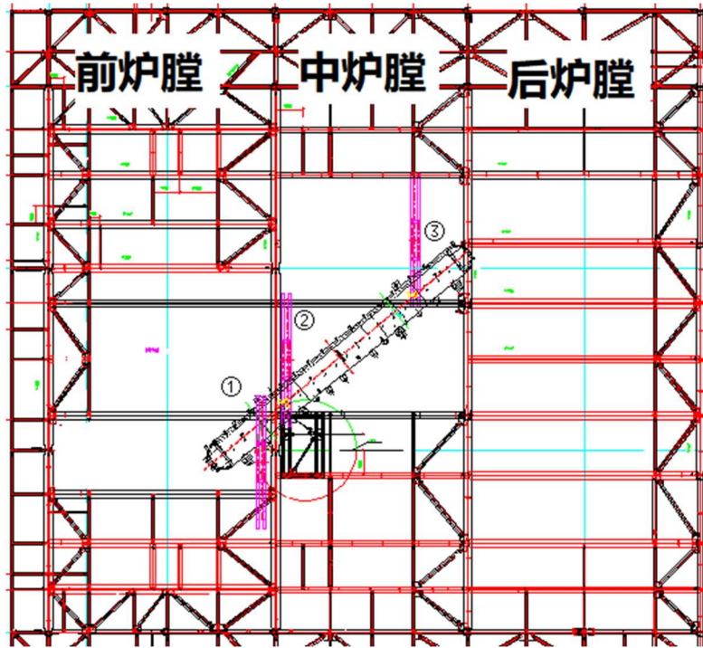
图6 汽包平移示意图-扩建端换钩
